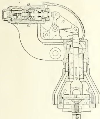
FIG. 5. VAPOR REGULATOR.
