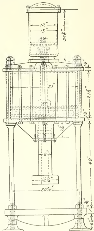
20-TON AIR PRESS
