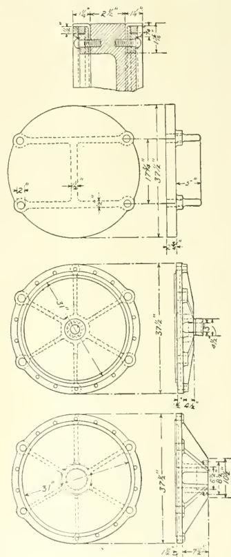
20-TON AIR PRESS
