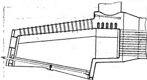
Millholland Boiler—1851.
