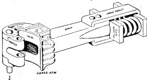
Couplers.—M. C. B. Type.
